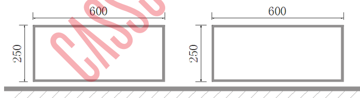
图 D.9 c) 平行式停车位车位线（单位：cm）
